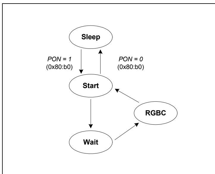
Figure 17: Simplified ALS State Machine
