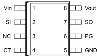
8-Pin SOIC (TPS7A69xx-Q1) D Package (Top View)
